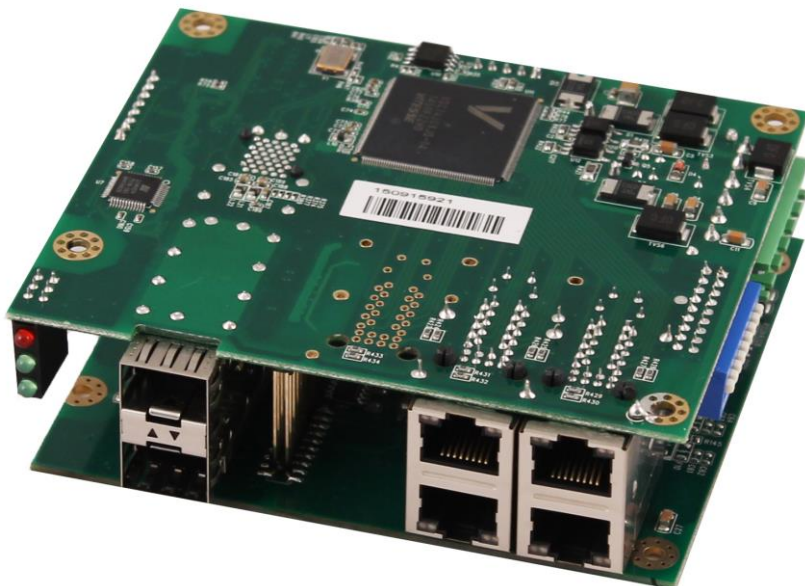
Рис.1 Коммутатор SW-60402/IC-P, внешний вид
