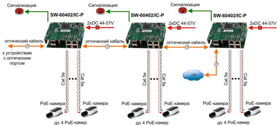
Рис.4 Типовая схема подключения коммутатора SW-60402/IC-P
