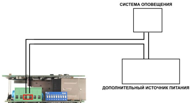
Рис.6 Схема подключения системы оповещения к коммутатору SW-60402/IC-P.
