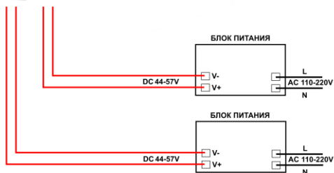
Рис.5 Схема подключения блоков питания к клеммной колодке коммутатора SW-60402/IC-P.
