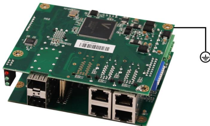
Рис.7 Заземление коммутатора SW-60402/IC-P
