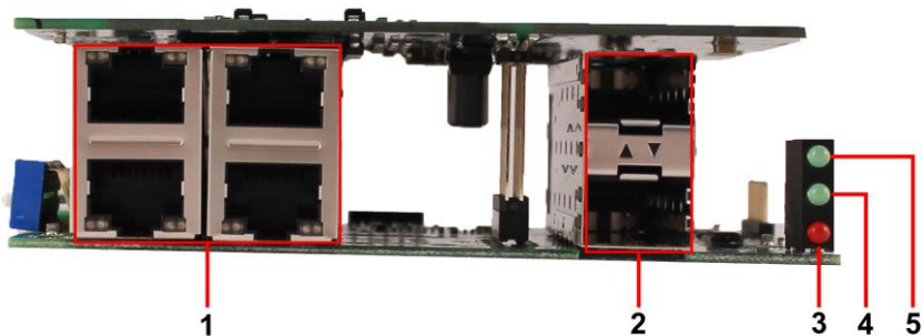
Рис. 2 Коммутатор SW-60402/IC-P, разъемы, кнопки и индикаторы, вид спереди.
