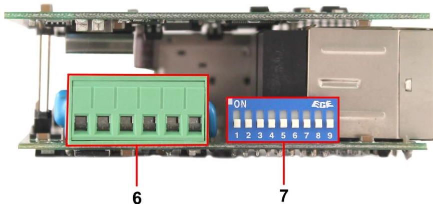
Рис. 3 Коммутатор SW-60402/IC-P, разъемы, кнопки и индикаторы, вид сбоку.
