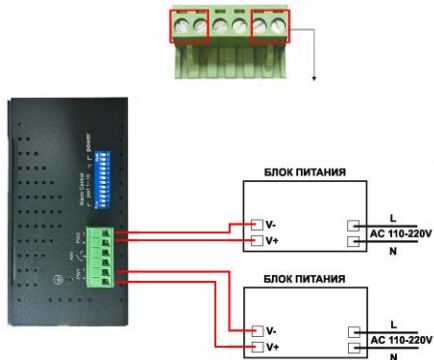
Рис.5 Схема подключения блоков питания к клеммной колодке коммутаторов SW-60822/ILC, SW-80822/ILC
