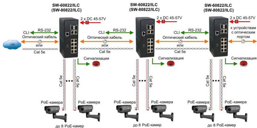
Рис.4 Типовая схема подключения коммутаторов SW-60822/ILC, SW-80822/ILC
