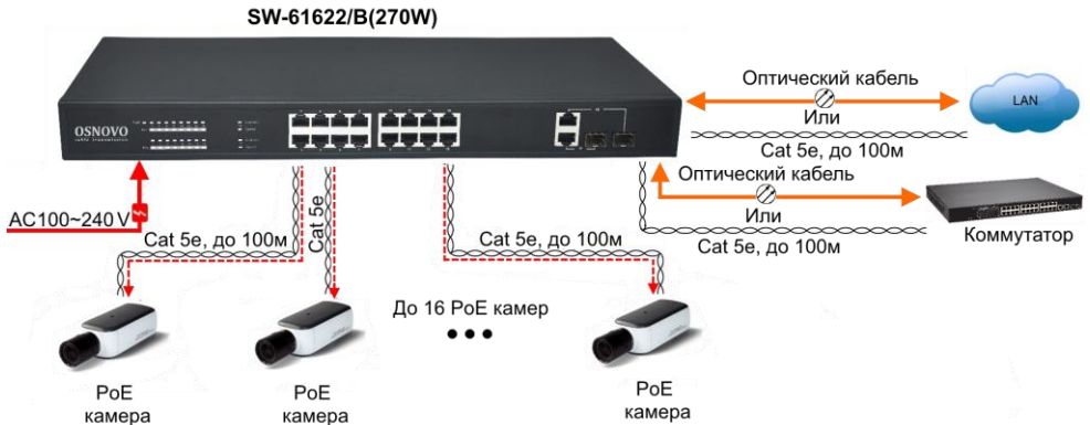
Рис.7 Типовая схема подключения коммутатора SW-61622/B(270W)
