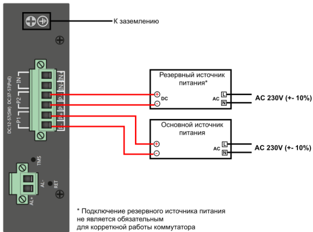
Рис. 10 Подключение блоков питания к коммутатору SW-80822/ILR
