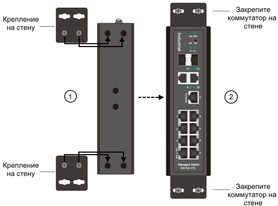
Рис. 13 Порядок монтажа коммутатора на стену
