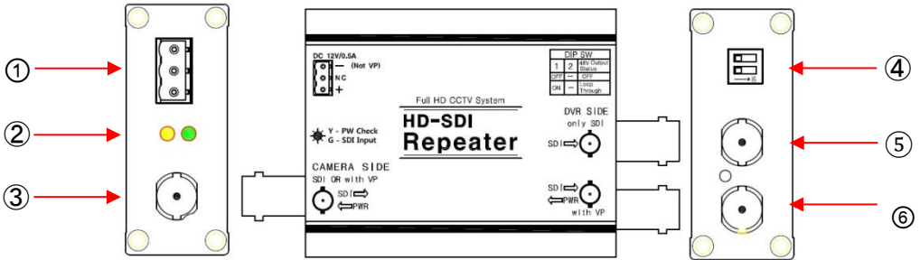
Рис. 6 Элементы E-SD12/P
