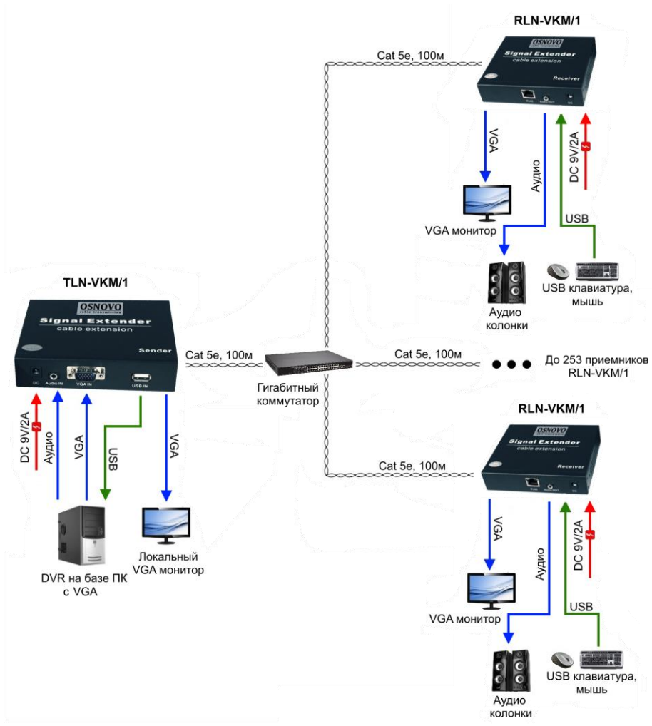
Рис. 6 Схема подключения комплекта TLN-VKM/1+RLN-VKM/1 через гигабитный коммутатор в режиме «точка-многоточка»
