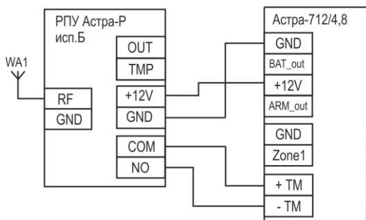
Рисунок А.1- Схема подключения «РПУ Астра-Р» исполнение Б
