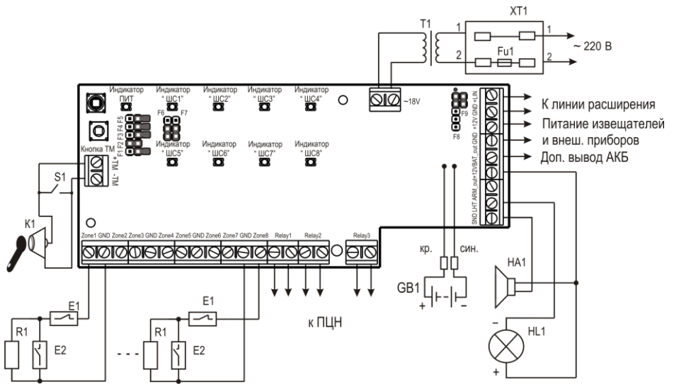
Рисунок А.2- Схема подключения извещателей, имеющих выход типа «сухой контакт» (релейный), и работающих на замыкание или размыкание
