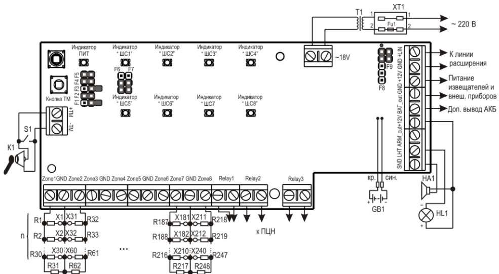
Рисунок А.3 - Схема подключения активных извещателей
