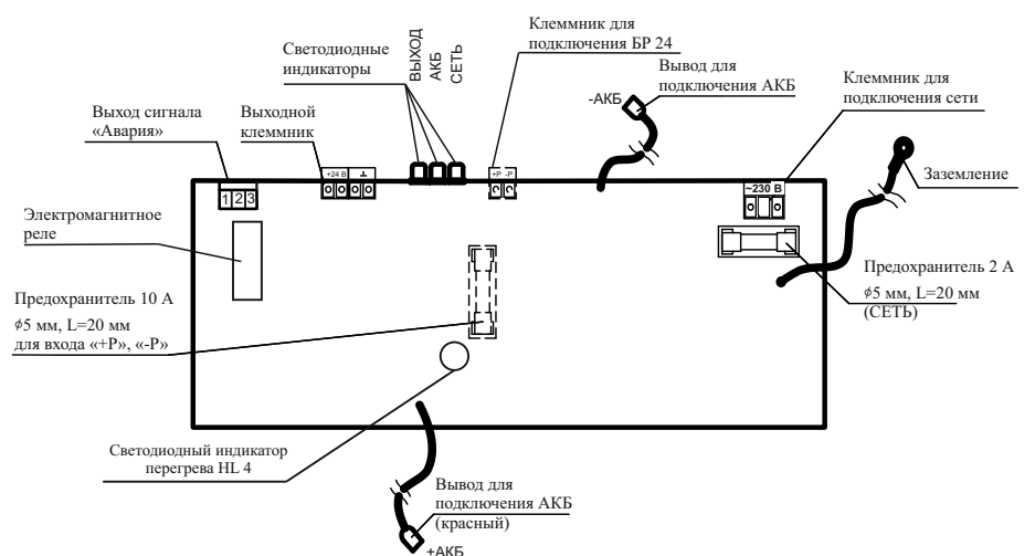
Рисунок 1 – Плата источника
